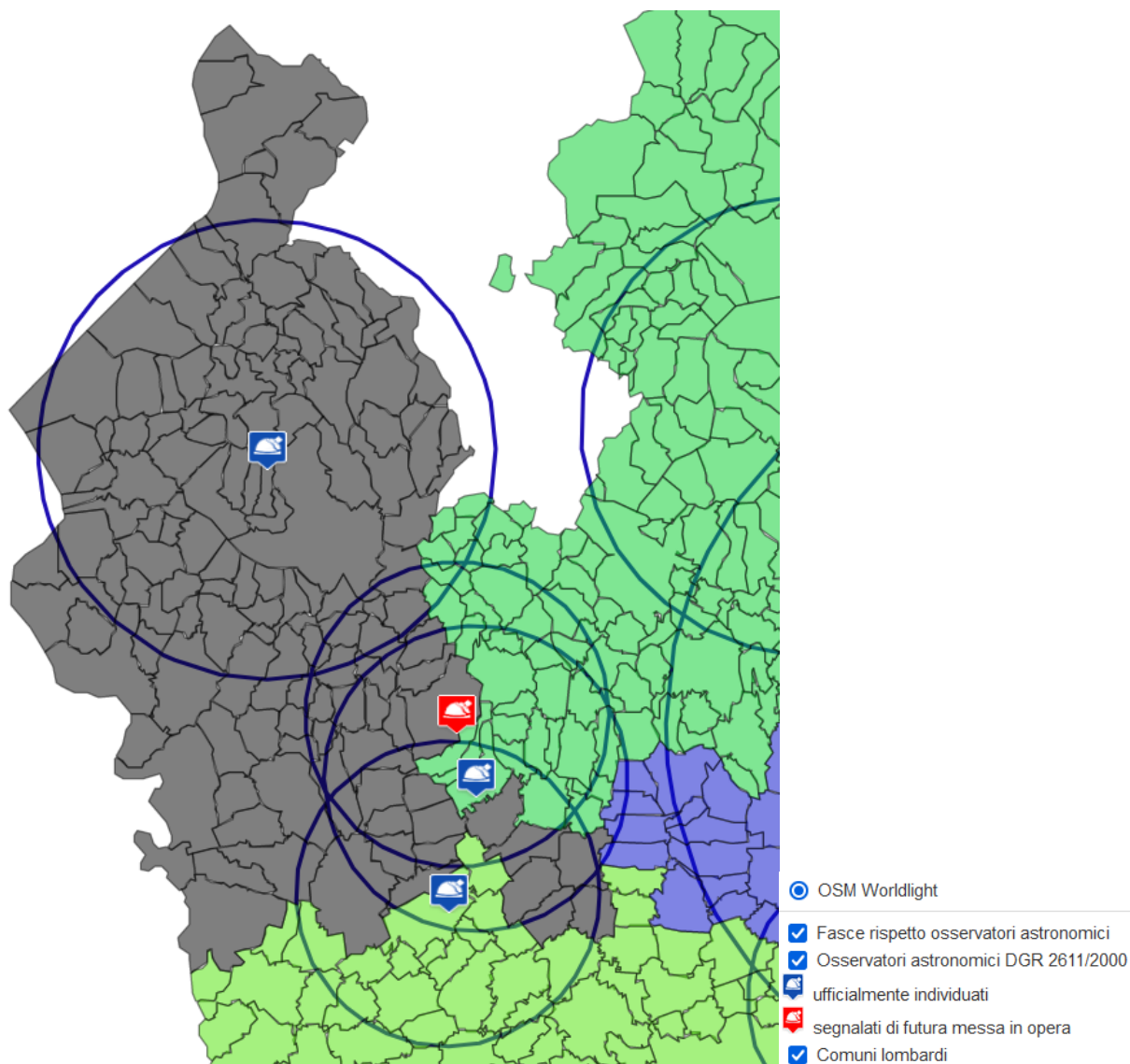
Figura 4.21 - Osservatori astronomici che interessano l'area del Parco
